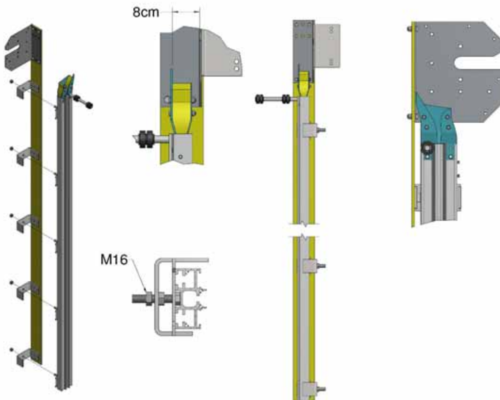
Abbildung 15, Schienenmontage
