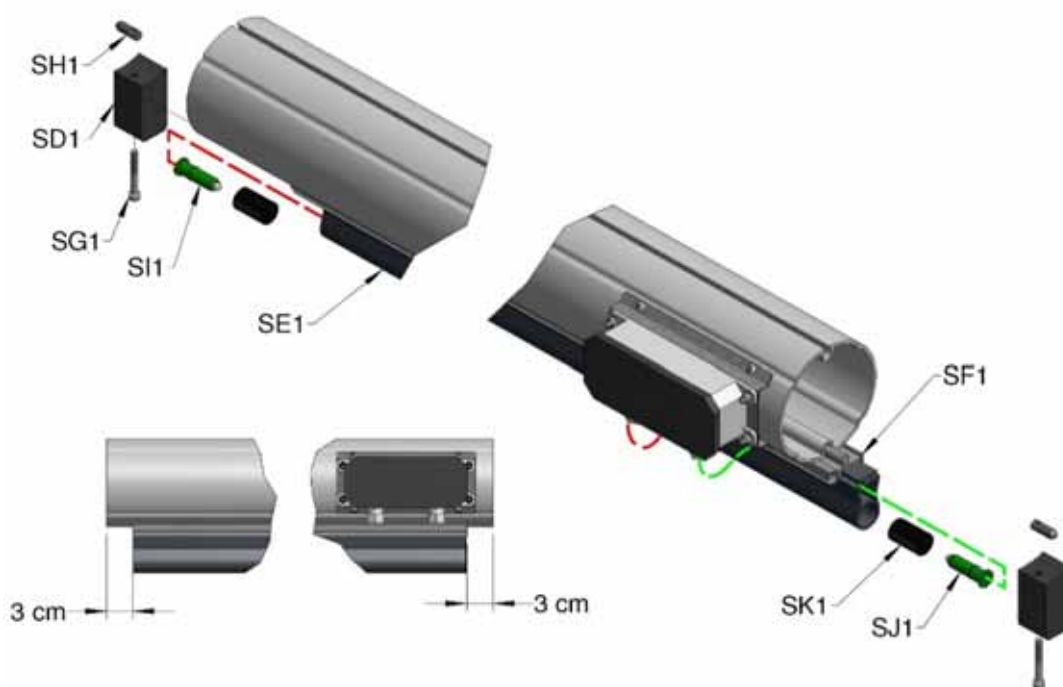
Abbildung 34b, Sicherheitskantenprofile
