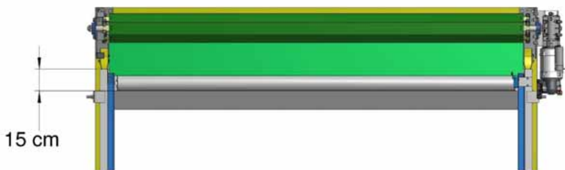
Abbildung 29, Grenzposition „Öffnen“
