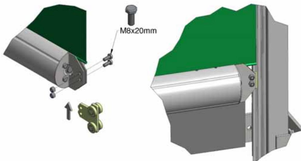
Abbildung 24, Anhang des unteren Laufrades
