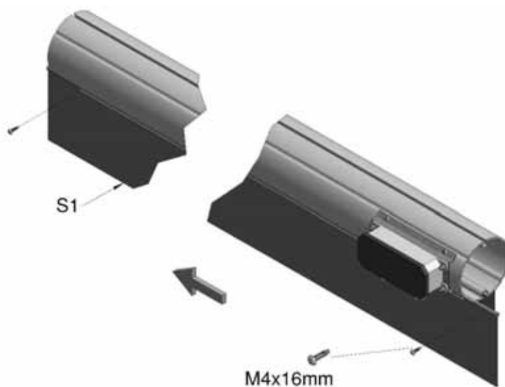
Abbildung 35, Untere Lasche
