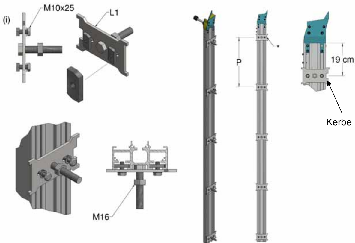
Abbildung 14: Schienenplatten-Baugruppe
