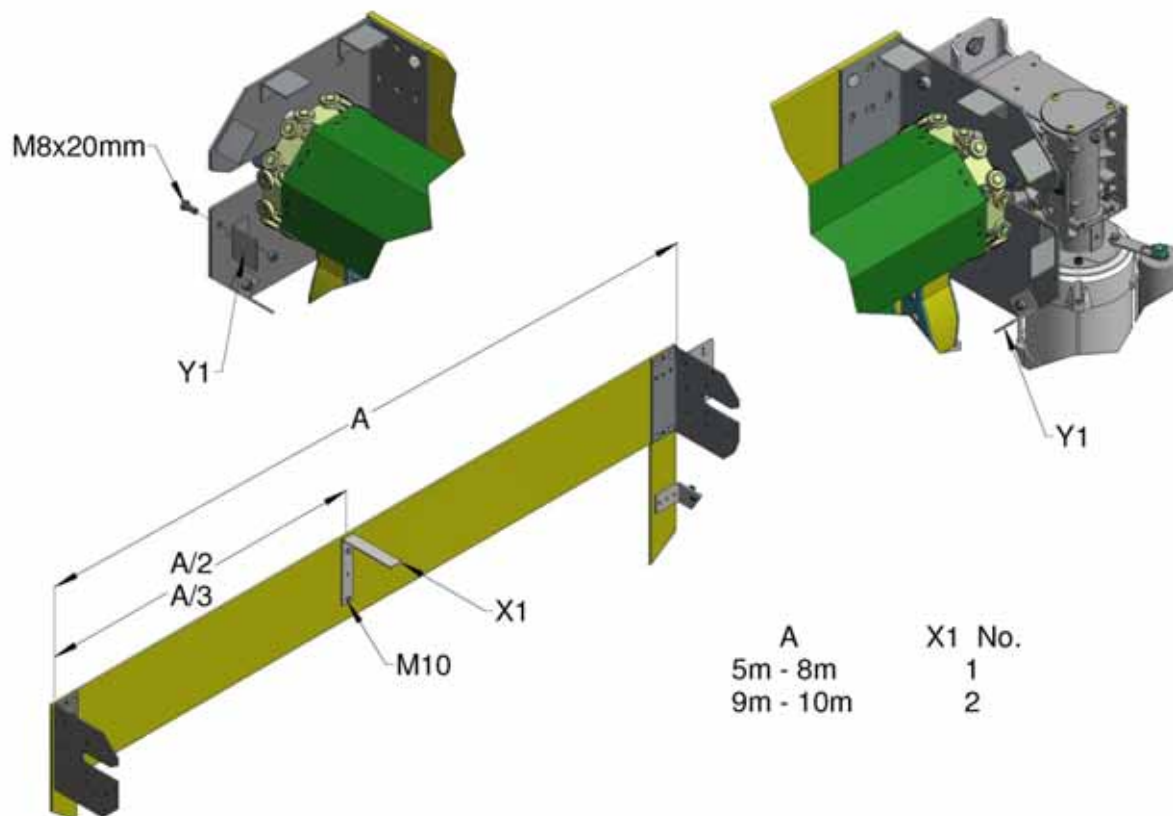
Abbildung 30: Abdeckblechhalterungen
