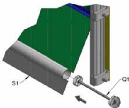
Abbildung 22, Untere Lasche und Rohreinsätze
