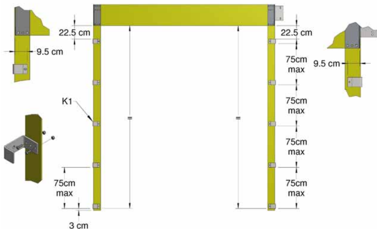
Abbildung 12, Schienenmontagehalterungen
