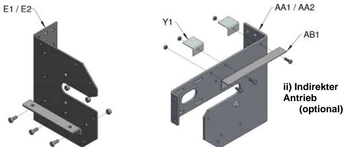
Abbildung 3, Motormontagehalterungen
