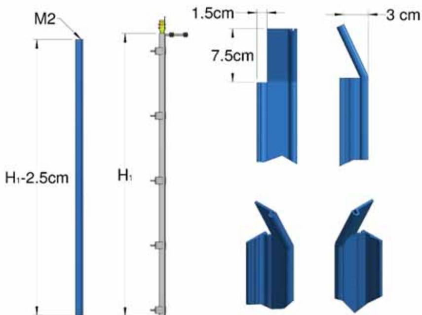
Abbildung 25a, Trennung der Schienenabdeckungsstreifen
