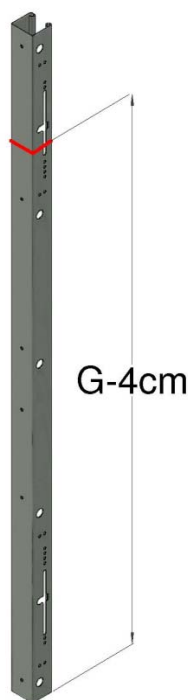
Figur 7, Sådan skæres styreskinnernes længder
