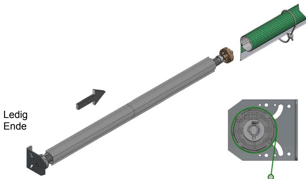
Figur 6b, Sæt fjedersamlingen ind i det øverste rør
